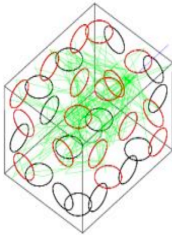
Scintillation
